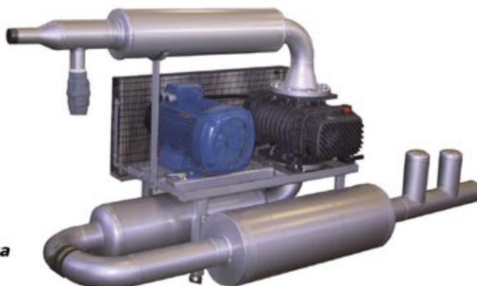
Depressore BORA 353 con silenziatori a risonanza
